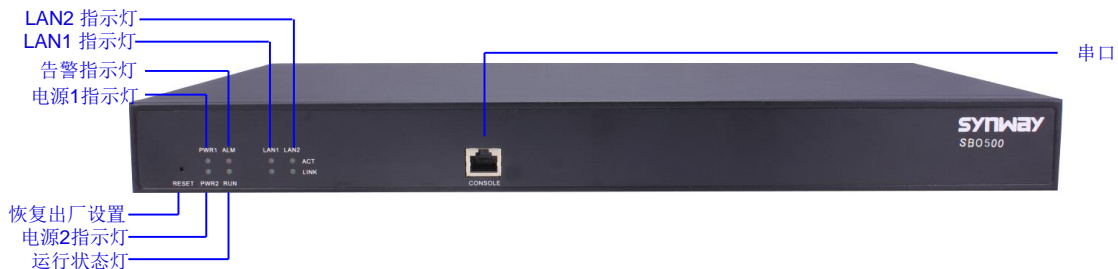
图 1-2 SBO500 前面板示意图
