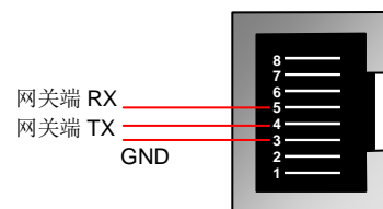
图 1-5 串口信号定义
