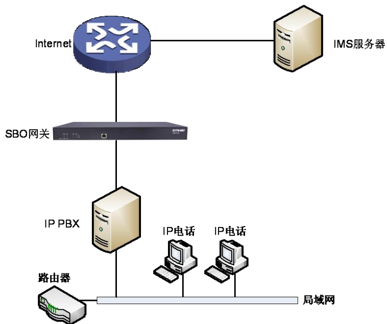
图 4-1 典型应用
